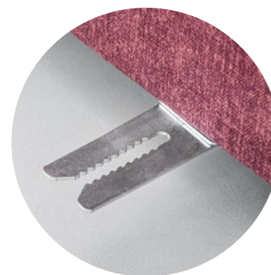
Verbinder zur Verbindung in Mehrpersonensets, unter dem Sockel montiert
